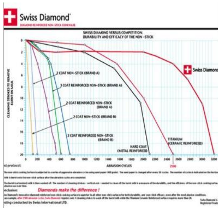
Diagramma di DURATA ed EFFICACIA del rivestimento AntiAderente.
